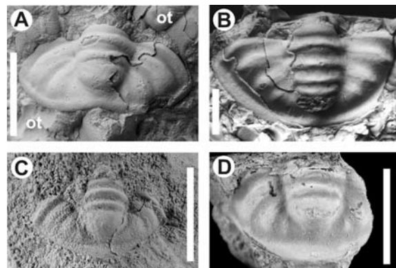
Text-fig. 23. Undetermined pygidia of exotic trilobites from the Furongian of Sweden. A – Pygidium indet. A, LO12091t, O. gibbosus or O. truncatus Zone at Övre Västerstad (Ö); B – Pygidium indet. B, LO12092t, O. gibbosus Zone at Övre Västerstad (Ö); C–D – Pygidium indet. C from the P. brevispina Zone at Hällekis (Vg). C – LO12093t; D – LO12094t. Accompanying fauna: ot – Olenus truncatus (Brünnich, 1781). Scale bars represent 0.5 cm
