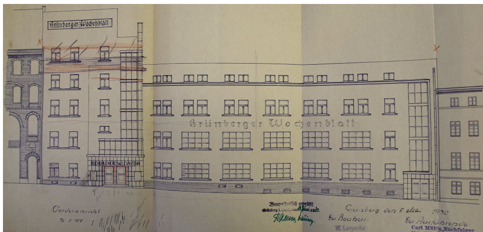
Fot. 3. Projekt budowlany nowej siedziby Tygodnika Zielonogórskiego” autorstwa Richarda Kintzla z 1930 roku
