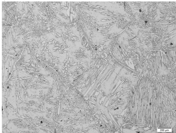
b) 0.024% C + 2.55% Cu
