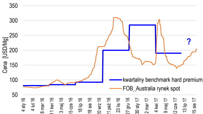
Rys. 4. Zmiany kwartalnych cen kontraktowych ( benchmark prices ) na tle indeksów cen na rynku spot dla węgla koksowego typu hard w latach 2016–2017
