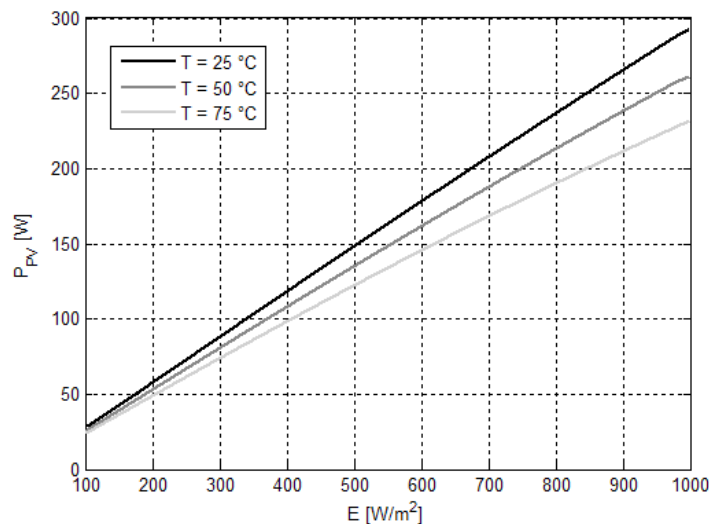
Rys. 6. Rodzina charakterystyk P_{PV} = f(E) modułu fotowoltaicznego
